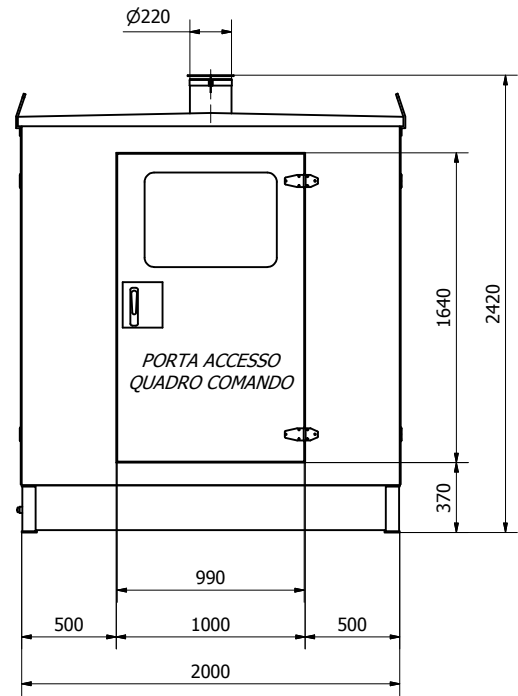
SCALA 1:40
